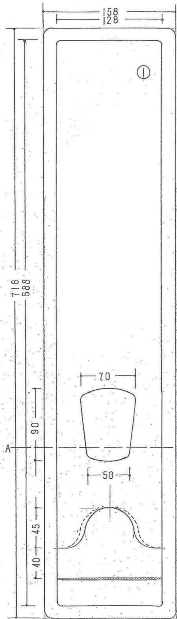
正面图
