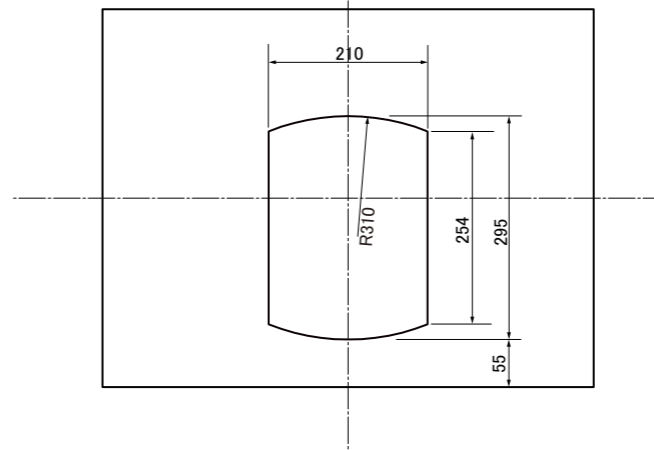
天板 開口図
