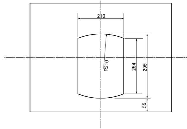
天板 開口図
